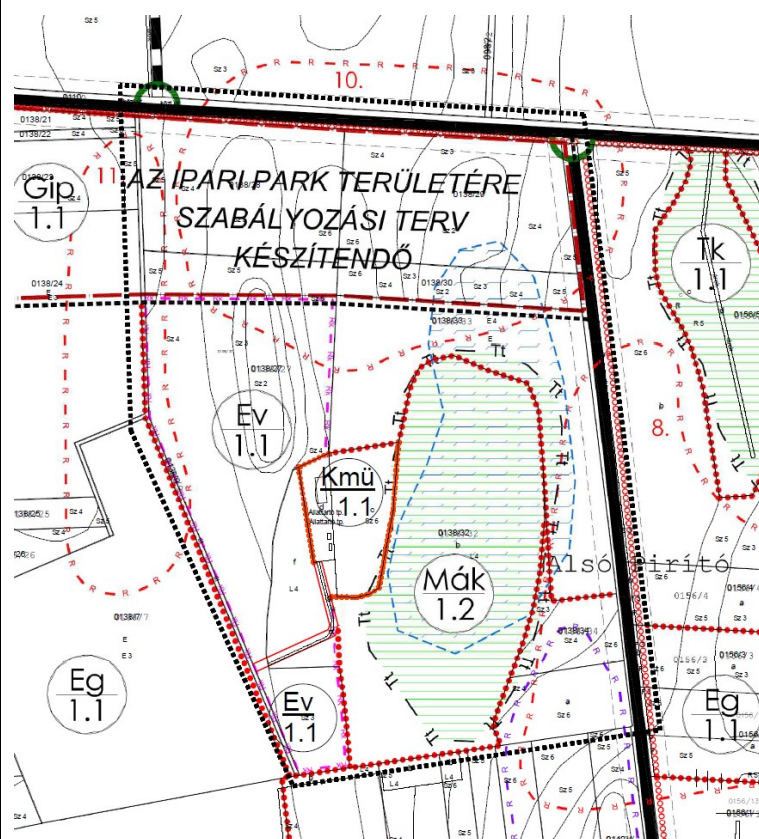
Tervezett állapot szabályozási terv
